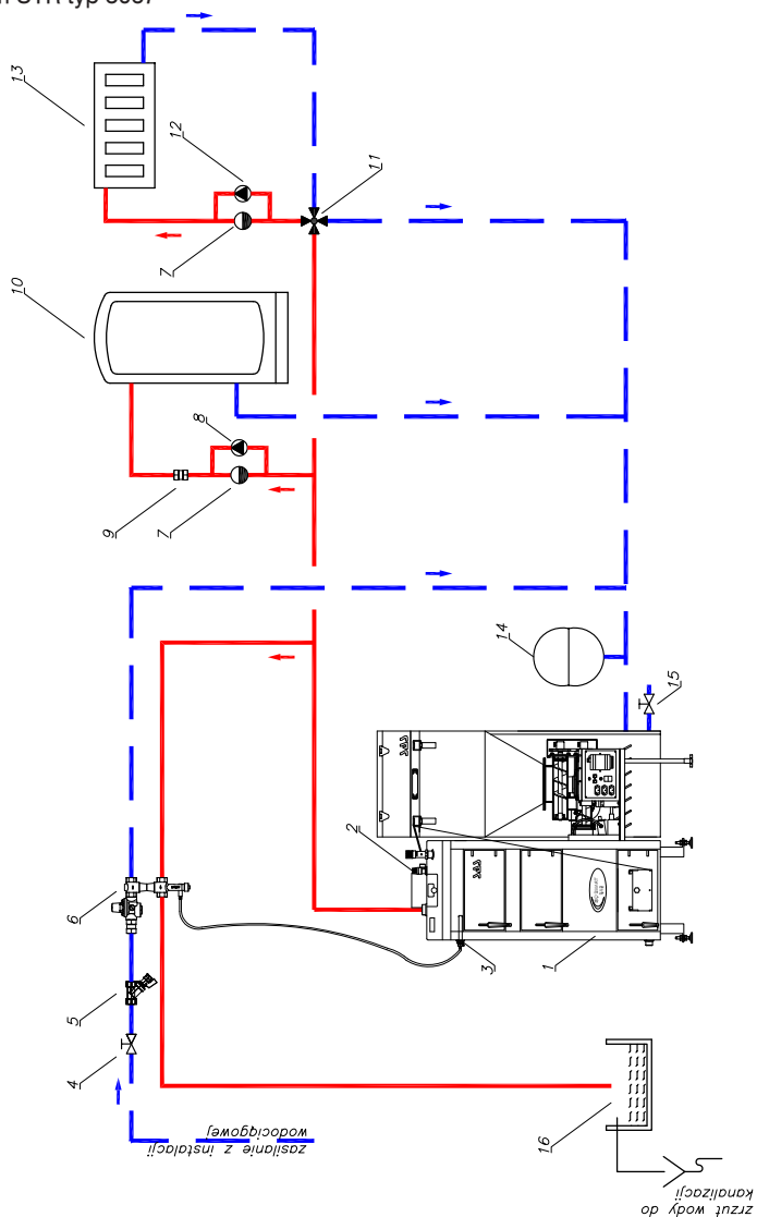
Rysunek.13. Schemat ogólny podłączenia kotła typu SAS BIO SMART do instalacji c.o. i c.w.u. Kocioł w układzie zamkniętym, zabezpieczony przed przegrzaniem zaworem termostaticznym SYR typ 5067
